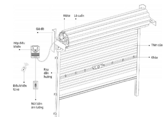
Mô hình lắp đặt
